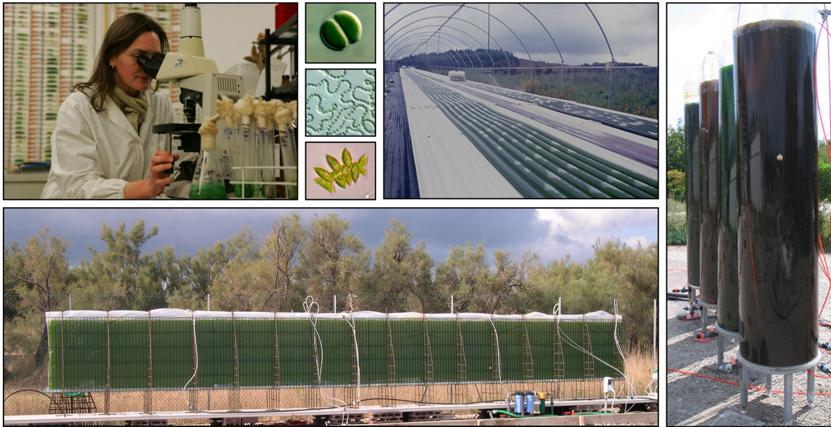
Figura 3- In alto a sinistra: parte della collezione di cianobatteri dell'ISE e del Dipartimento di Biotecnologie Agrarie. In basso ed a destra: fotobioreattori per colture algali massive progettati dai ricercatori del Dipartimento di Biotecnologie Agrarie di Firenze e commercializzati da F&M srl ( www.femonline.it ).
