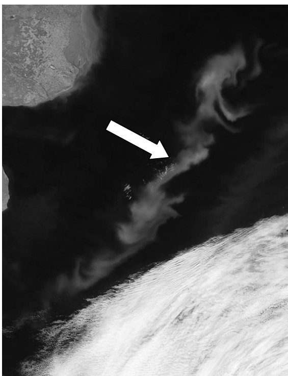
Figura 1 - Bloom algale al largo delle coste argentine ( http://oceancolor.gsfc.nasa.gov/SeaWiFS/ )
