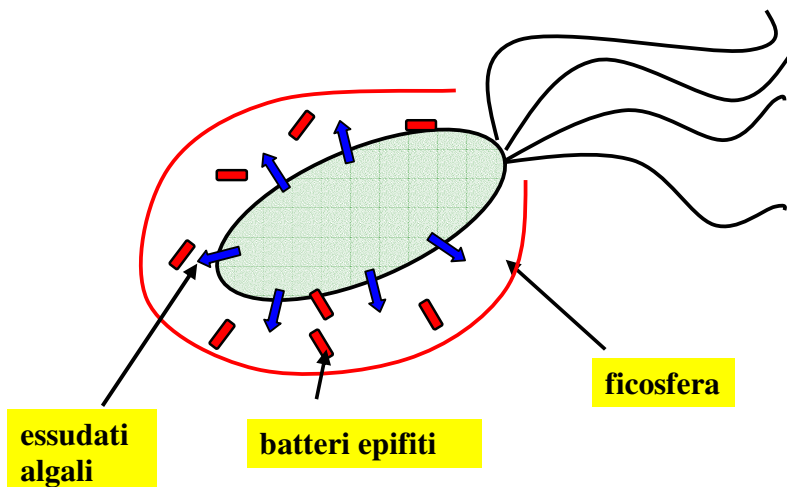
Figura 4 - La ficosfera. Le microalghe rilasciano sostanze (essudati) che favoriscono lo sviluppo dei batteri epifiti che a loro volta producono sostanze stimolanti la crescita algale.
